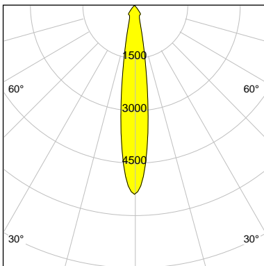
I-max : 5409 cd/klm
