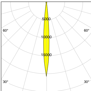
I-max : 20741 cd/klm
