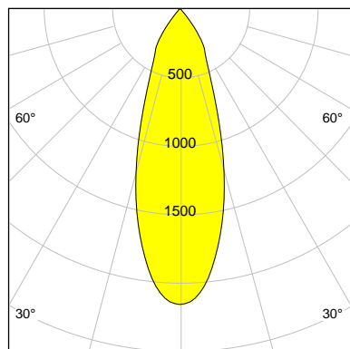
I-max : 2162 cd/klm
