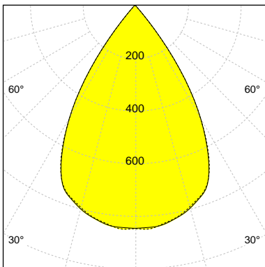
I-max : 852 cd/klm
